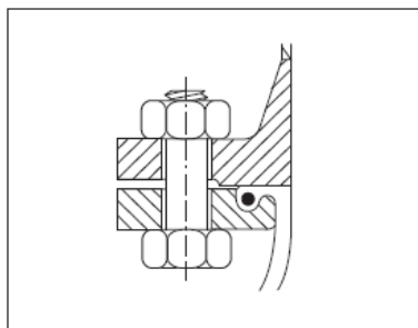
Fig. 2 Brides dotées d'une surface d'appui lisse.
