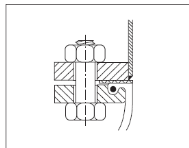
Fig. 4 Brides fournies avec joint plat servant à protéger la surface en caoutchouc.
